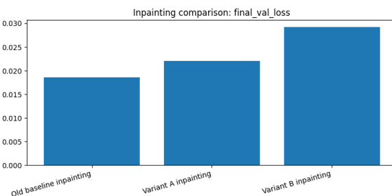
5(d) Validation loss
